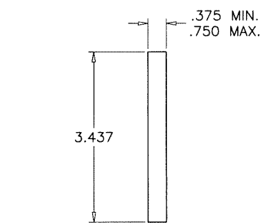
6 SIDE BAR
